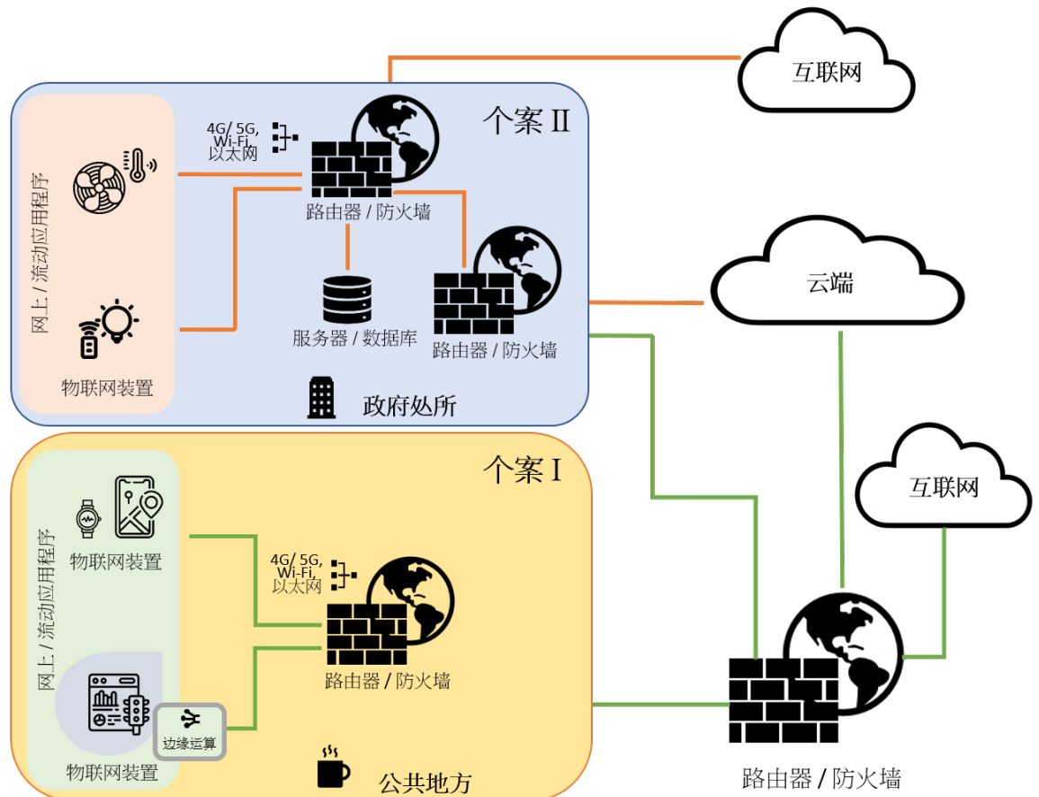
图 7.1 宏观物联网参考模型
